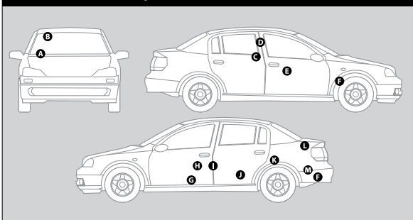
Gráfica para Ubicación de Placa de Identificación de Partes de Servicio para Vehículos de General Motors
