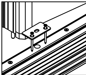
Figura 2e (Umbral de balanceo interno)
