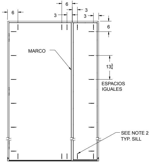
PUERTA ÚNICA CON LISTONES (CHS)
