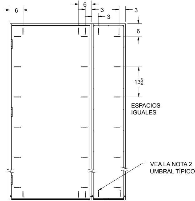
PUERTA ÚNICA CON LISTONES (EN CAJA)
