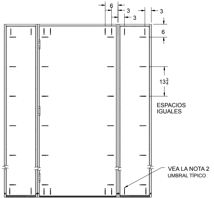
PUERTA ÚNICA CON LISTONES (EN CAJA)
