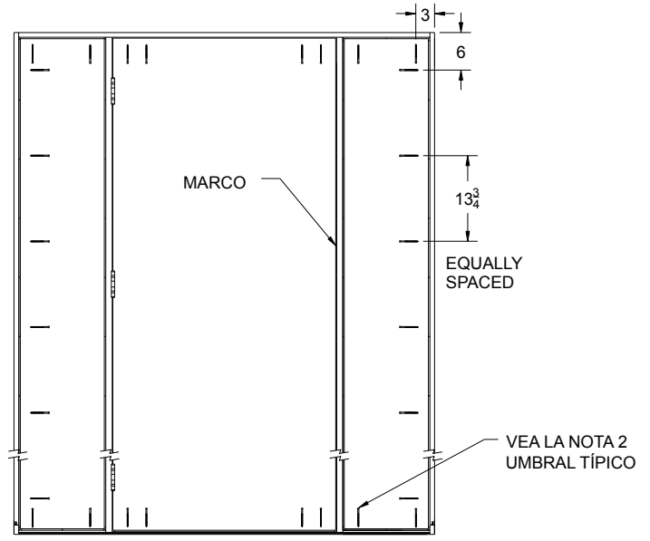
PUERTA ÚNICA CON LISTONES (CHS)
