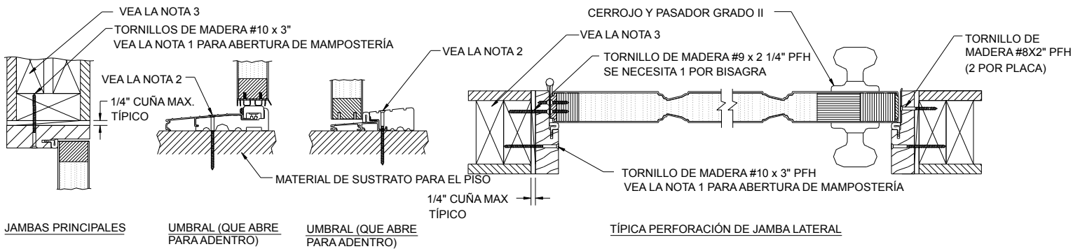
PUERTA ÚNICA CON LISTONES (EN CAJA)
