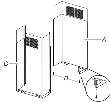
A. Assemblage de la partie supérieure et de la partie inférieure du cache-conduit - (placement à l'avant) B. Chevilles en plastique (2) (extrémité longue pour placement à l'avant) C. Assemblage de la partie supérieure et de la partie inférieure des cache-conduits - (placement à l'arrière)
